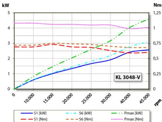
Leistungsdigramm Flüssigkeitsgekühlt
