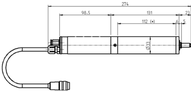
寸法図
