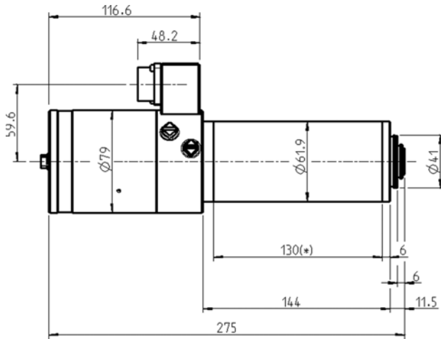
寸法図
