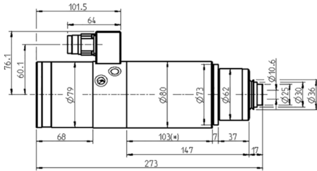
尺寸
