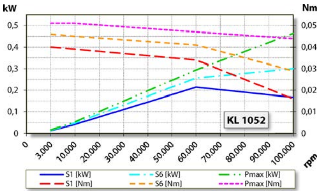
功率图
