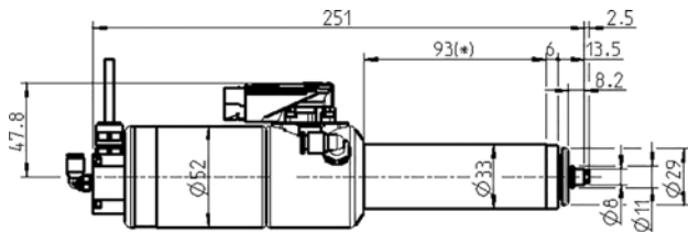
Abmessungen
